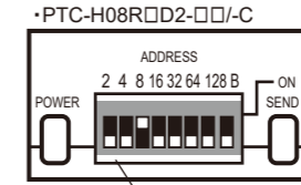
アドレス設定スイッチ 上向き設定でONです。
