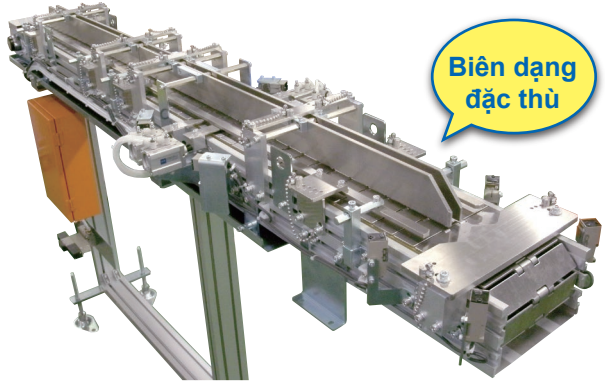
Con lăn dẫn hướng
