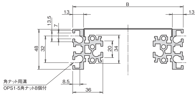
フレーム断面
