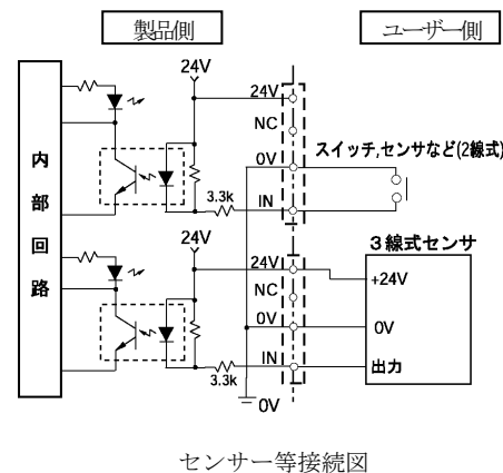
センサー等接続図
