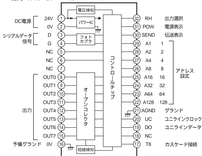
出力マスタモジュール SAP-H08
