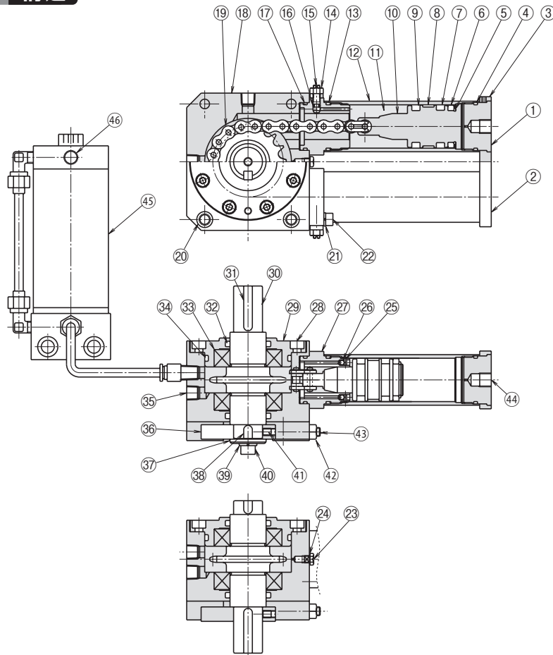
U型(下軸タイプ)
