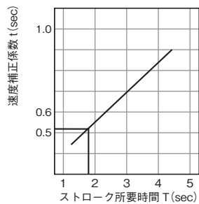
●グラフ6-7 NSB40-700(水平)
